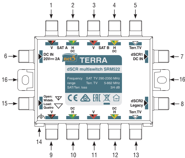
Рис. 1. Внешний вид мультисвича
